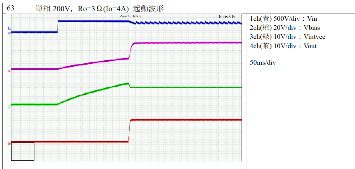
図 8-11 起動波形 [単相 200V, I_{out}=4A ]
