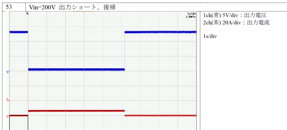
図 8-13 短絡試験[单相 200V]
