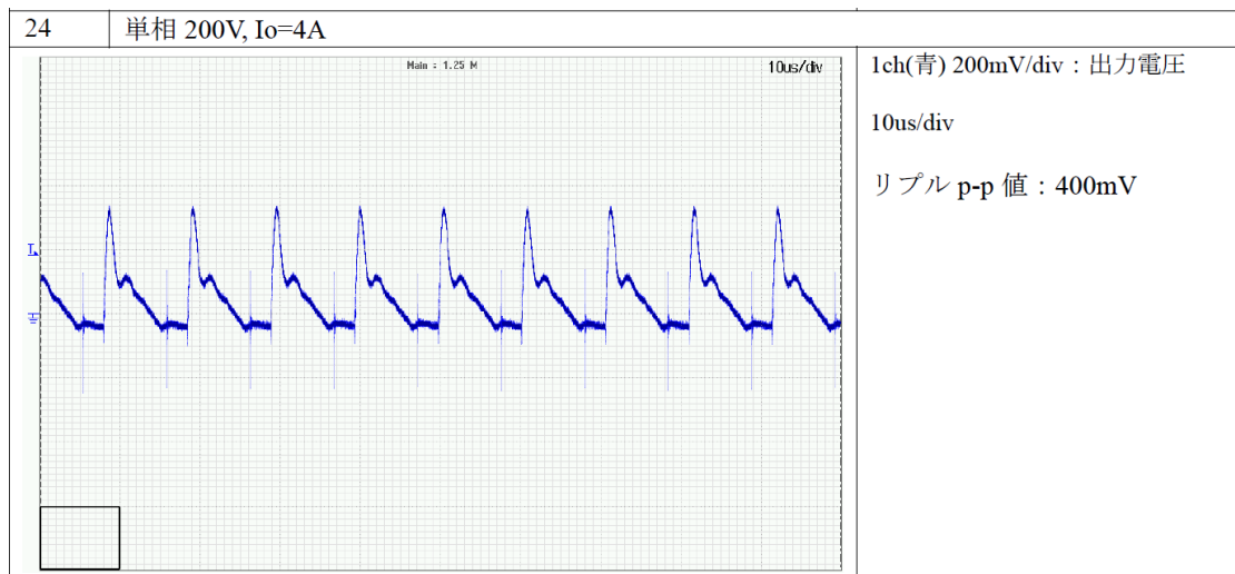
図 8-4 リプル特性 [单相:200V, I out =4A]
