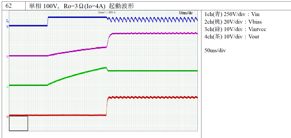
図 8-10 起動波形 [単相 100V, I_{out}=4A ]
