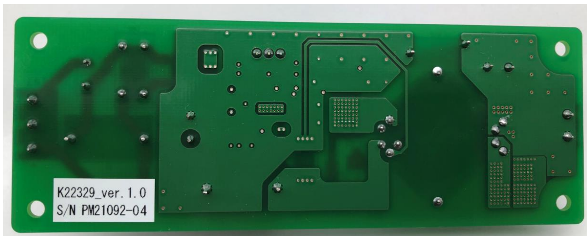
5-4 基板部品面写真(B 面)
