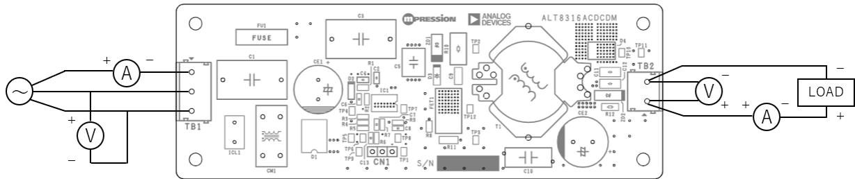
図 7-1 測定回路
