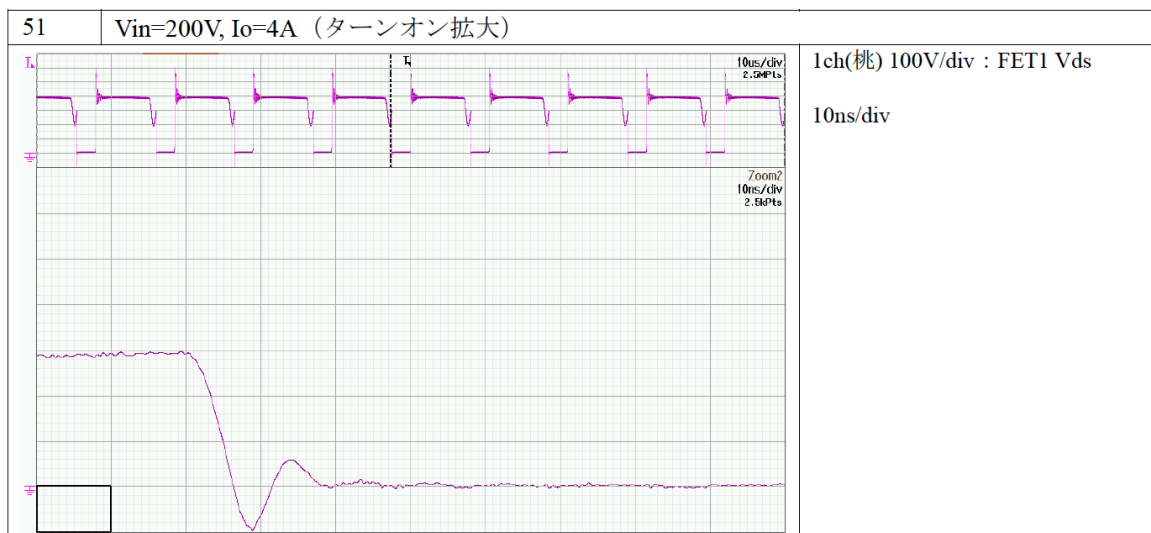
図 8-9 スイッチング波形 [単相 200V, Iout=4A(ターンオン波形)]
