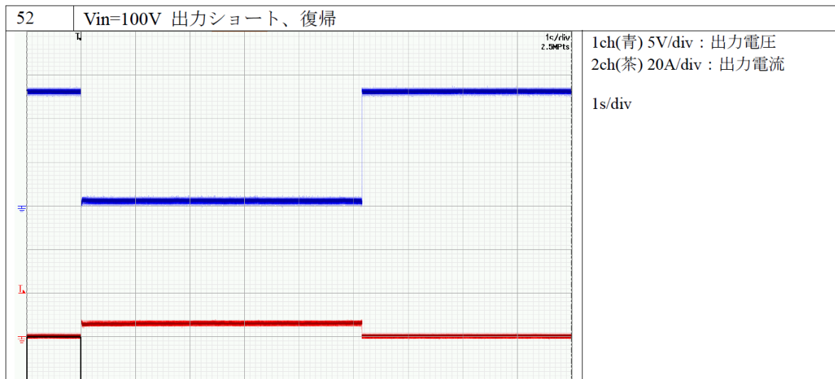
図 8-12 短絡試験[单相 100V]
