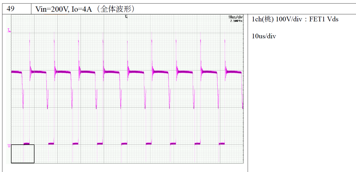
図 8-7 スイッチング波形 [単相 200V, Iout=4A(全体波形)]
