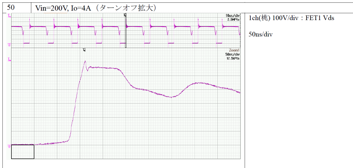
図 8-8 スイッチング波形 [単相 200V, Iout=4A(ターンオフ波形)]
