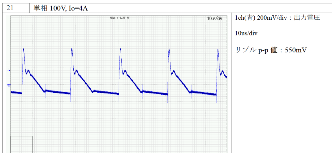
図 8-3 リップル特性 [単相:100V, Iout=4A]
