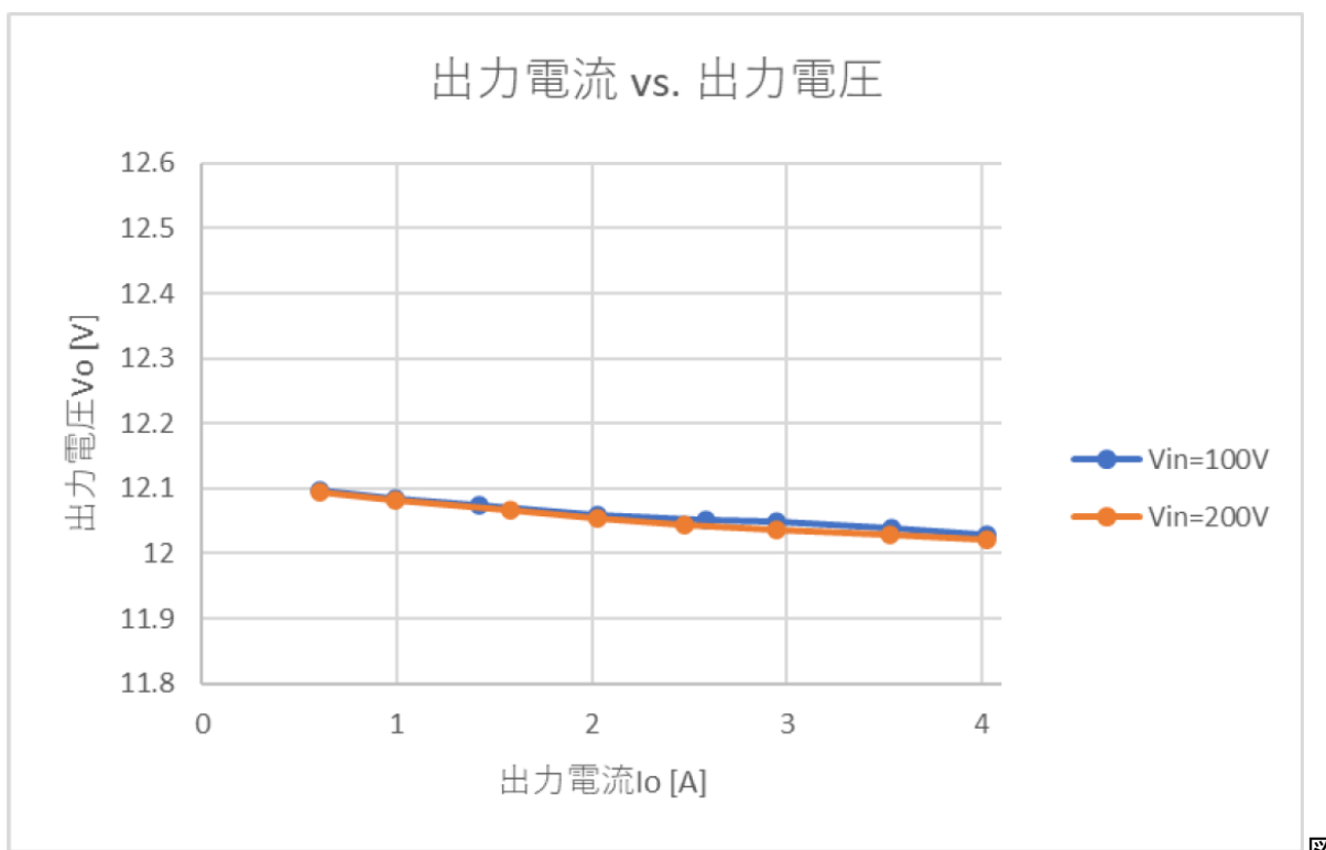
8-1 出力特性
