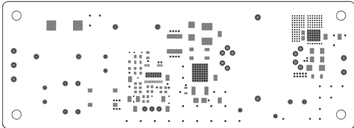
図 5-2 基板部品面(B 面)
