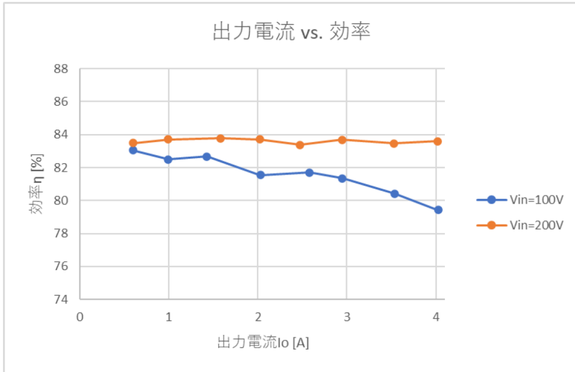
図 8-2 効率特性
