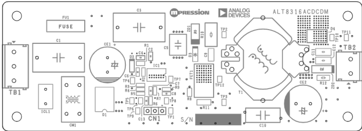
図 5-1 基板部品面(A 面)
