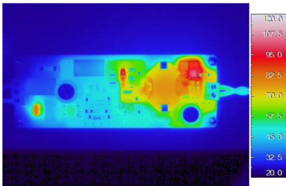
図 8-16 サーモグラフィー画像[单相 200V]
