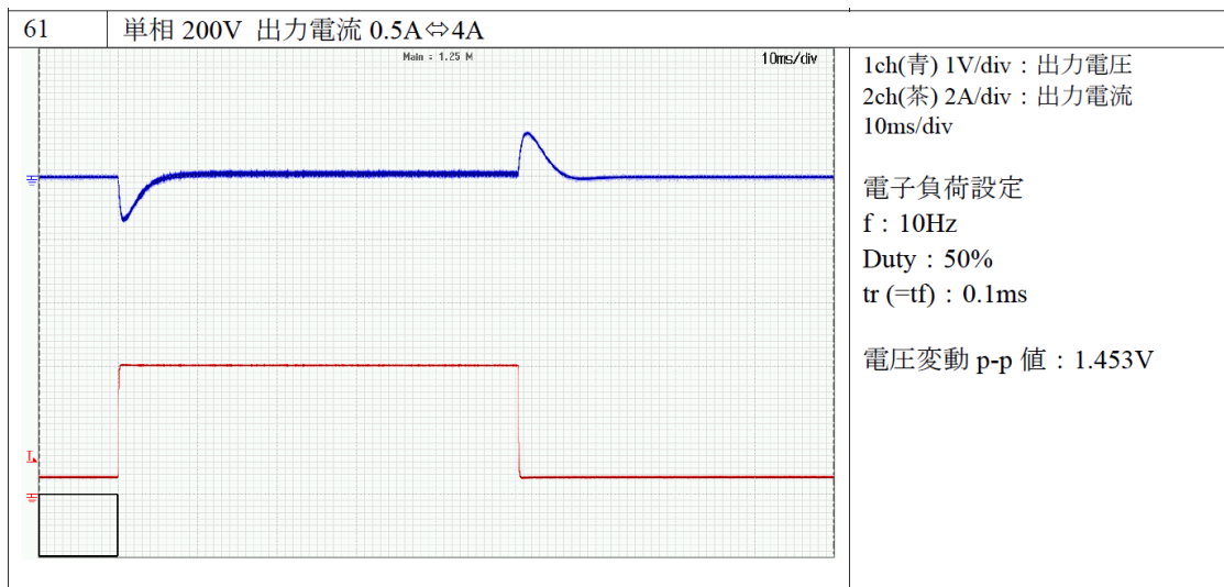
図 8-6 負荷応答性 [単相 200V, Iout:0.5A⇔4A]
