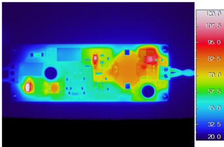
図 8-15 サーモグラフィー画像[单相 100V]
