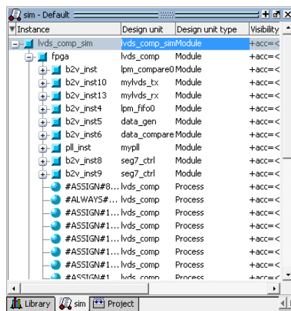
図 3-5-3 sim ウィンドウ例
