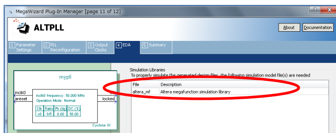
図 3-4-2 メガファンクションのライブラリ確認(例:PLL)
