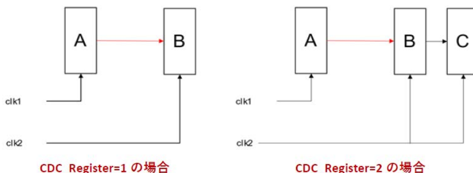
図 5-26. CDC_register アトリビュートの適用イメージ
