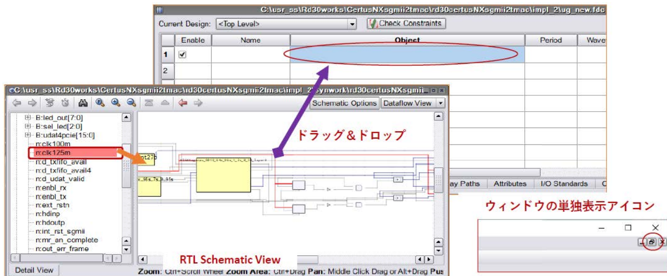
図 5-15. オブジェクトのドラッグ&ドロップとウィンドウの個別表示アイコン（右下）
