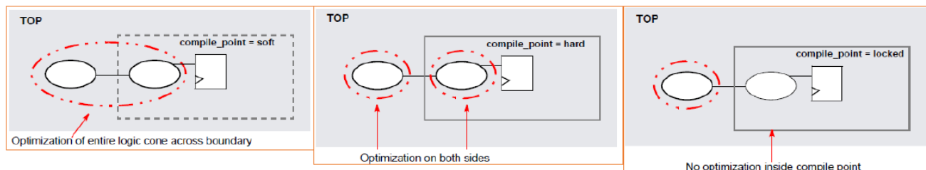
図 5-16. コンパイルポイント・タイプによる最適化の違い
