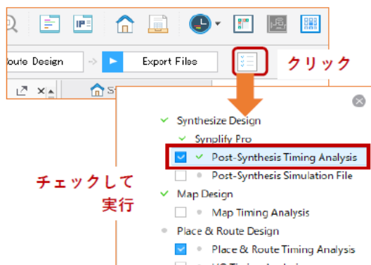
図 5-25. 論理合成プロセスのタイミング・レポート
