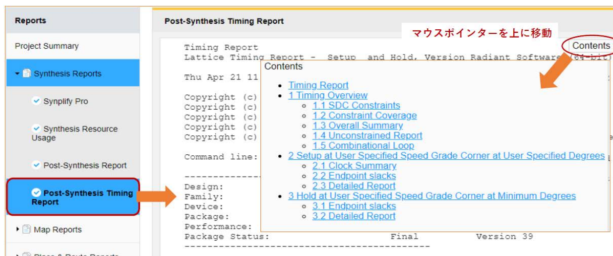
図 5-25. 論理合成プロセスのタイミング・レポート
