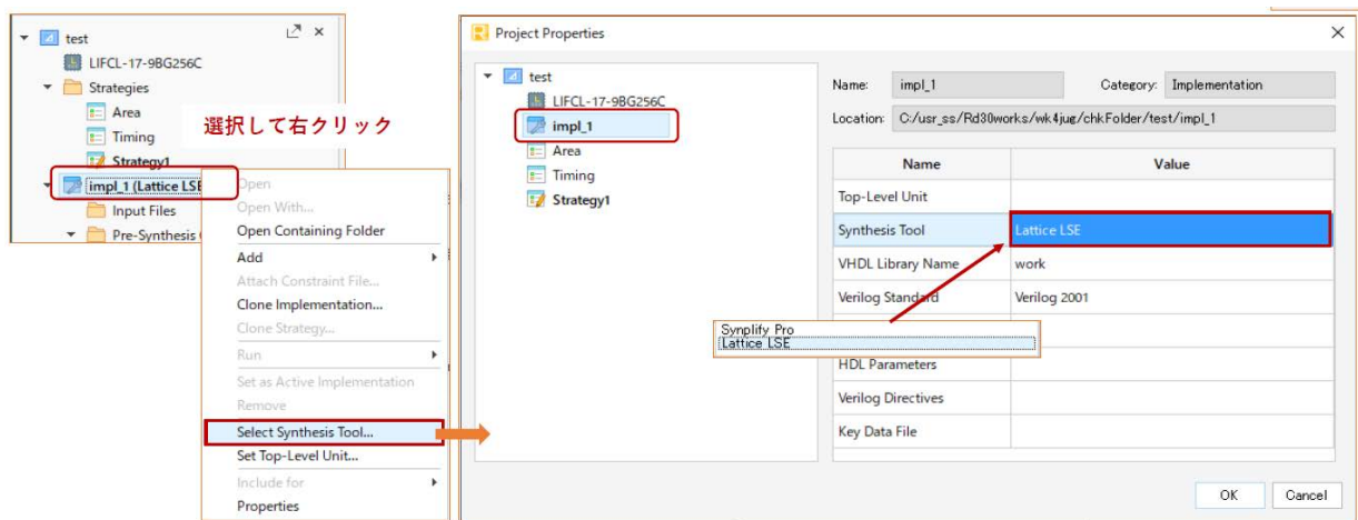
図 5-1. 論理合成ツールの変更操作 1
