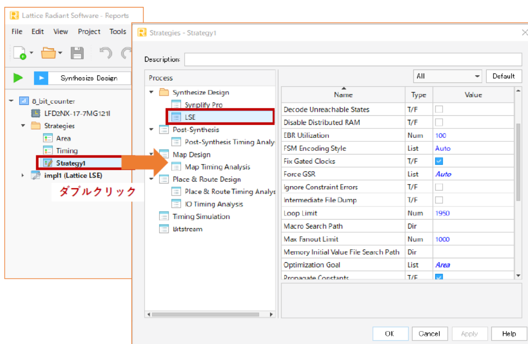
図 5-5. LSE のストラテジー設定ウィンドウ
