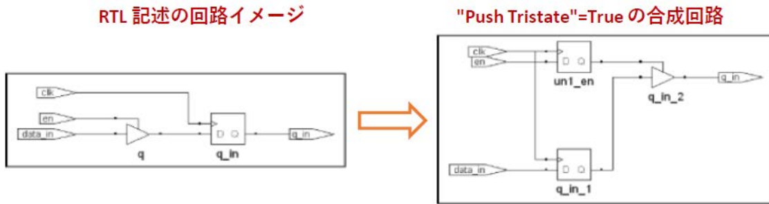
図 5-9. Push Tristate オプションの作用
