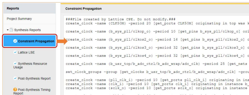
図 5-21. 制約プロパゲーション・レポート
