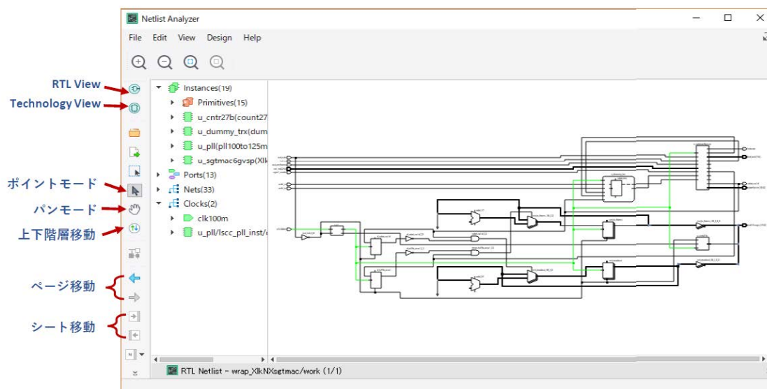
図 5-6. ネットリスト・アナライザーの表示例とアイコン
