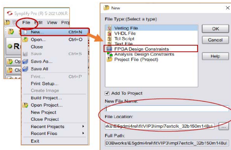
図 5-11. SCOPE エディタの起動
