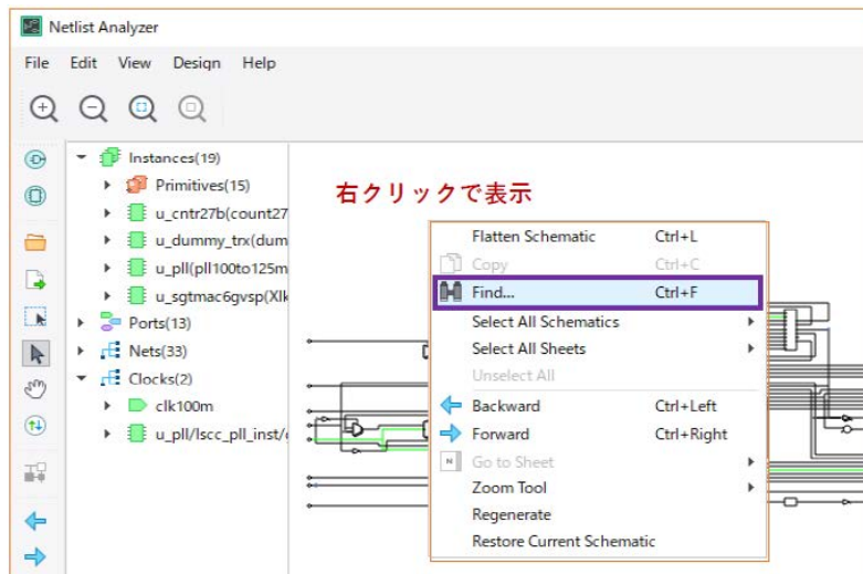
図 5-8. Find Dialog ウィンドウ
