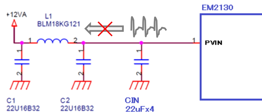
参考回路
